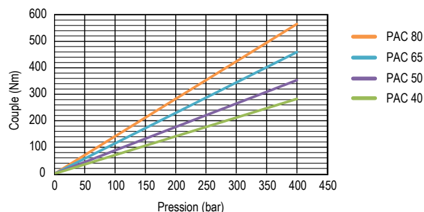
Modèles simple débit PAC
